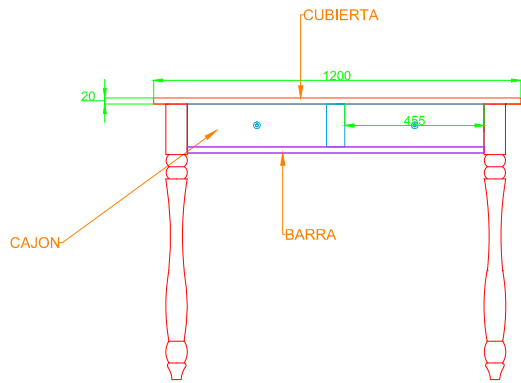
elevacion frontal
